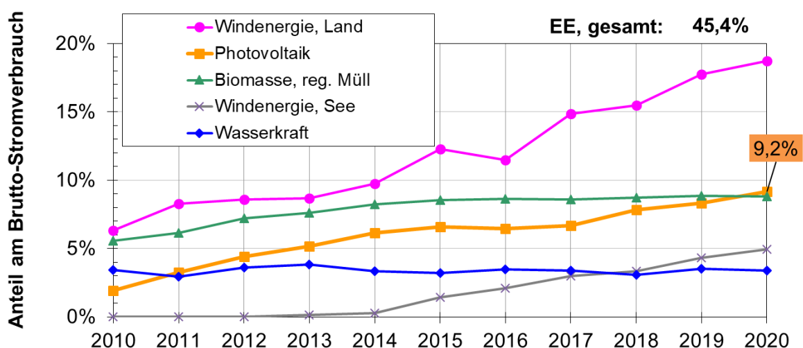
Abbildung 2: Entwicklung des Anteils Erneuerbarer Energien am Brutto-Stromverbrauch in Deutschland, Daten aus [BMW1], [UBA1], [ISE4]
