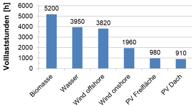
Abbildung 36: Prognostizierte Vollbenutzungsstunden für Stromerzeugung aus EE, Daten aus [ÜNB]
