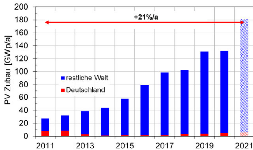
Abbildung 44: Entwicklung des jährlichen PV-Zubaus für Deutschland und die restliche Welt, Zahlen von EPIA, IHS, Solar Power Europe, mit Prognose für 2021.
