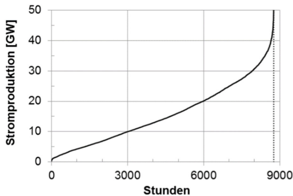
Abbildung 26: Stromproduktion PV + Wind in aufsteigend geordneten Stundenwerten für das Jahr 2017, Daten aus [ISE4]
