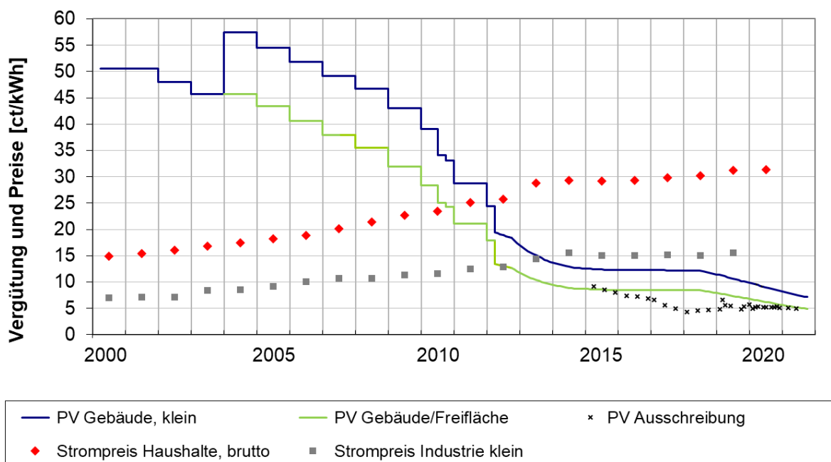
Abbildung 5: EEG-Vergütung für PV-Strom nach dem Datum der Inbetriebnahme des Kraftwerks, mittlere Vergütung in den Ausschreibungen der Bundesnetzagentur, Strompreise, Daten aus [BMW1], [BDEW6]
