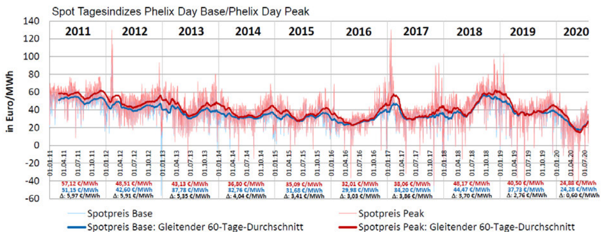
Abbildung 6: Strompreisentwicklung am Day-Ahead Spotmarkt [BDEW6]
