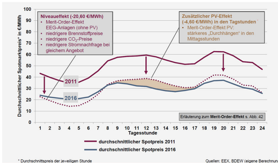
Abbildung 8: Einfluss von EE auf die durchschnittlichen Spotpreise an der Strombörse [BDEW2]
