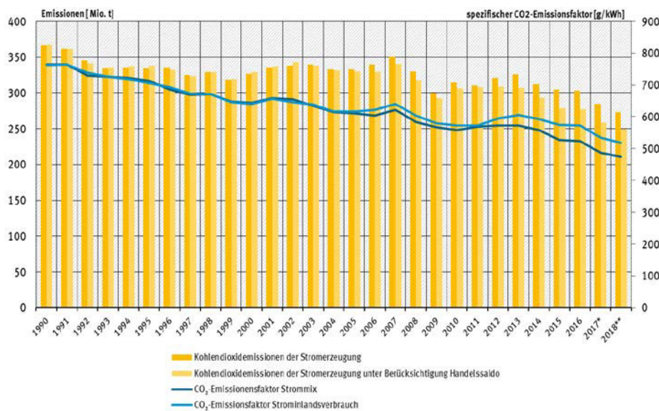
Abbildung 42: Spezifische und absolute CO 2 -Emissionen der Stromerzeugung in Deutschland [UBA6]
