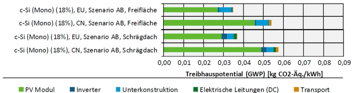
Abbildung 40: Treibhauspotential der Stromerzeugung mit mono c-Si PV für Dach- und Freiflächenanlagen [UBA7]
