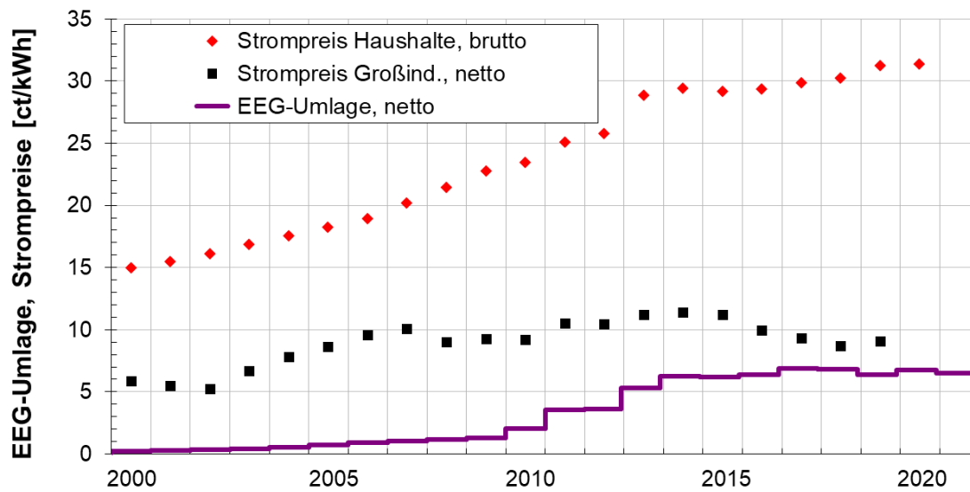
Abbildung 14: Entwicklung von Brutto-Strompreisen für Haushalte, von Netto-Strompreisen für industrielle Großabnehmer und Entwicklung der EEG-Umlage, Daten aus [BMW1]
