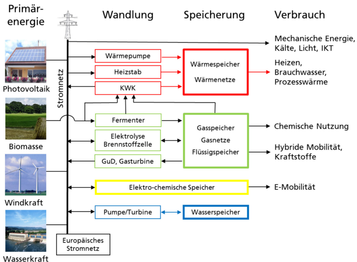
Abbildung 62: Vereinfachte schematische Darstellung eines Erneuerbaren Energiesystems mit den wichtigsten stromnetzgebundenen Bausteinen der Gewinnung, Wandlung, Speicherung und des Verbrauchs
