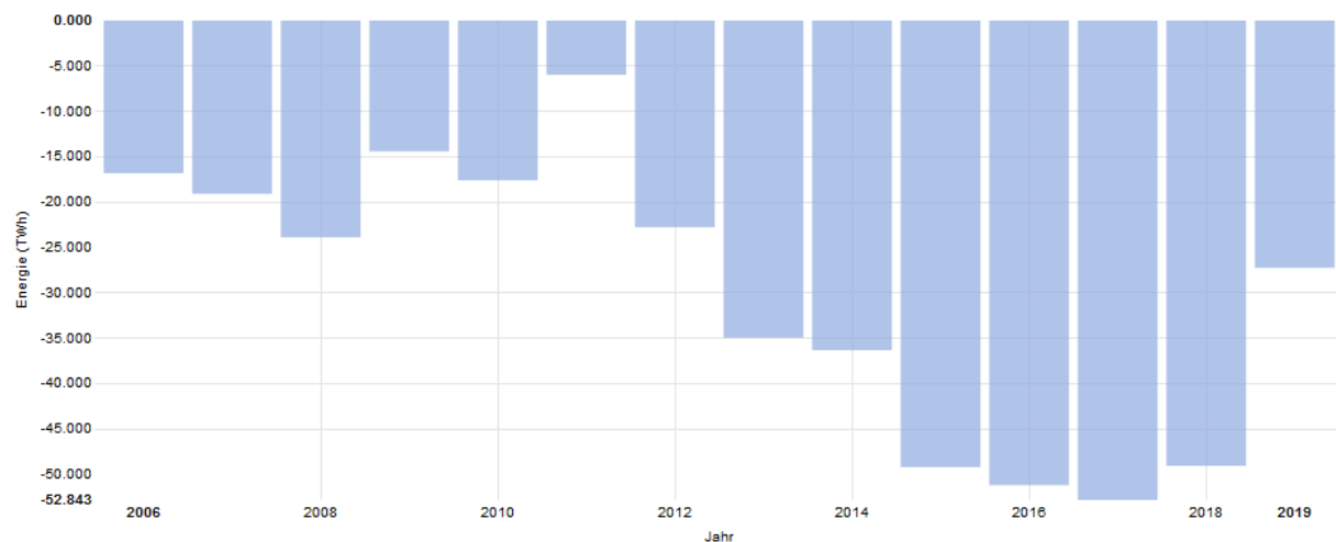
Abbildung 16: Stromexport (als negative Werte) für Deutschland [ISE4]
