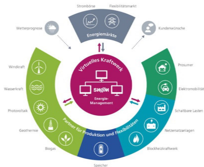
Abbildung 20: Konzept für ein virtuelles Kraftwerk der Stadtwerke München [SWM]
