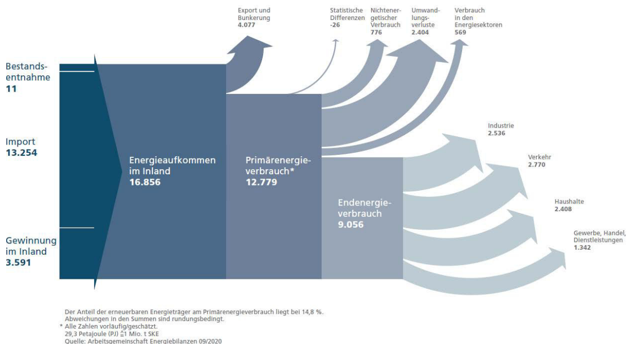
Abbildung 45: Energieflussbild 2019 für Deutschland, Angaben in Petajoule [AGEB]
