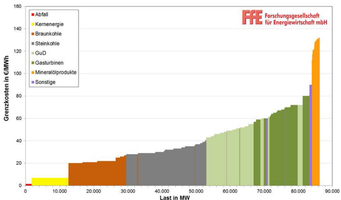
Abbildung 7: Merit Order konventioneller Kraftwerke im Jahr 2018 bei einem mittleren CO 2 -Zertifikatspreis von 16 €/t [FFE]
